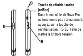
Vue latérale
